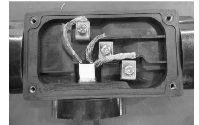
Cable1
