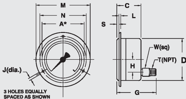
LBM/FRONT FLANGE
