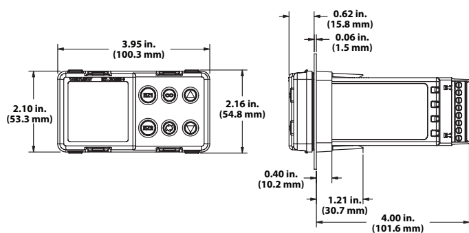
EZ-ZONE PM 1/8 DIN - Horizontal
